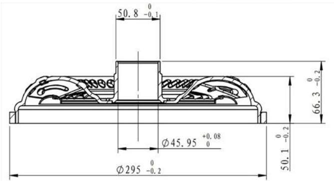
被测工件尺寸图
